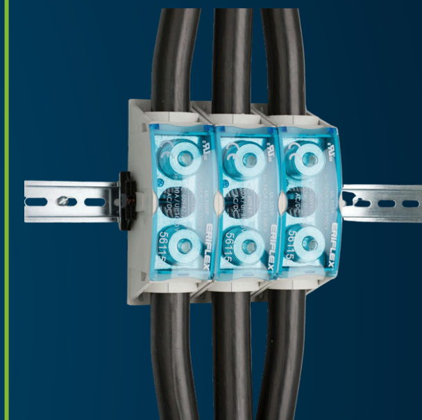
BLOCS DE DISTRIBUTION ET ALIMENTATION
